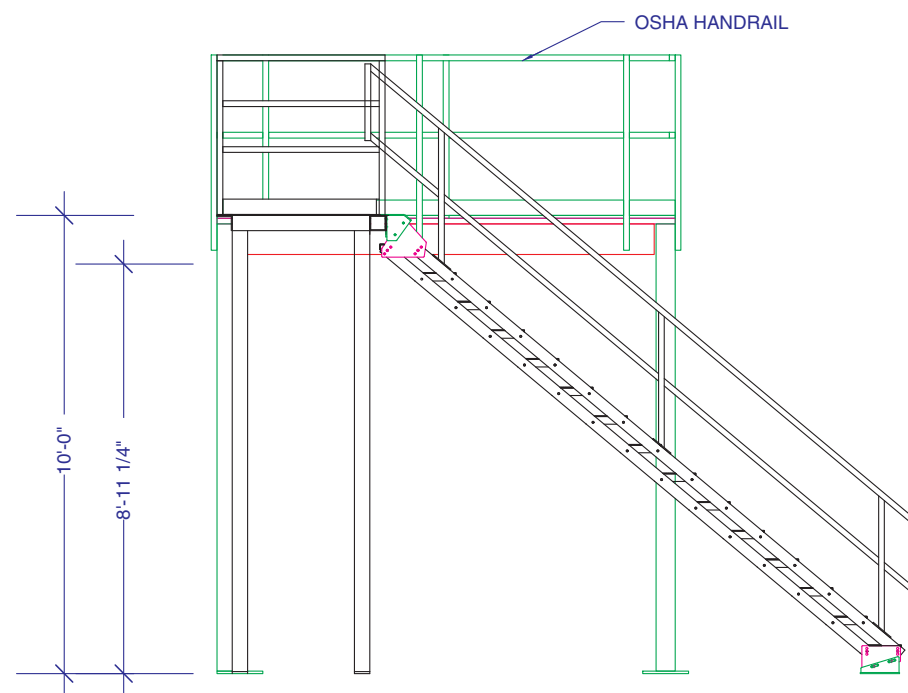
ELEVATION
